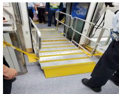
〔改良型横取りブリッジ〕
