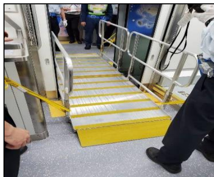
〔改良型横取りブリッジ〕
